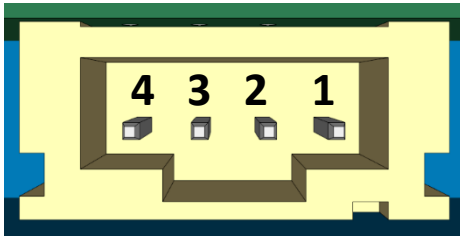
Şekil 1b: VE.Direct iletişim bağlantı noktasının pin numaralandırması.
