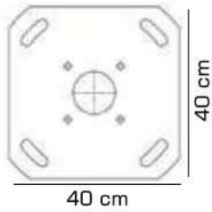
ANKARAJ BOYUTLARI Anchorage dimensions
